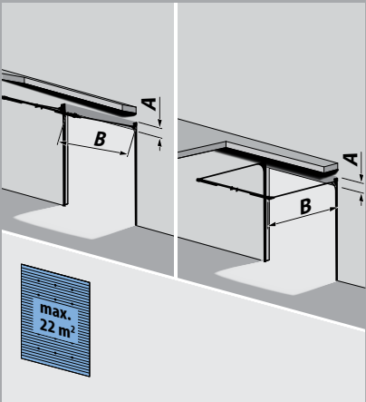
T 340 (B34), système de rails normal, arbre-ressort arrière + profilé de support en acier
