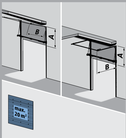
T 400 hF (B350), système de rails levée semi-verticale avec axe de ressort surbaissé + profilé de support en acier
