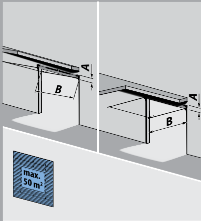
T 450 (B45), système de rails normal (standard)
