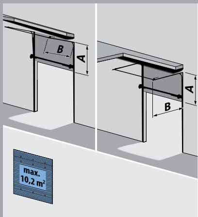
T 400 DS (B350 dock), système de rails levée semi-verticale avec axe de ressort surbaissé
