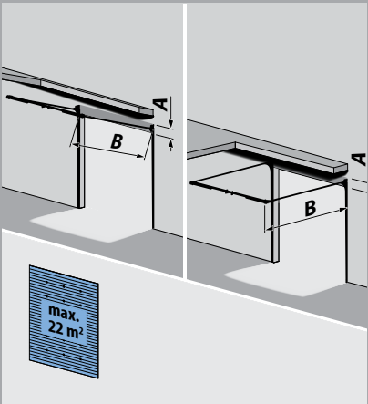
T 240 (B24), système de rails à linteau réduit, câbles glissés à l'intérieur + profilé de support en acier
