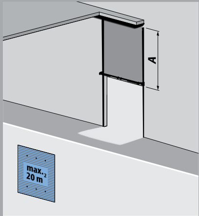
T 500 hF (B550), système de rails vertical avec axe de ressort surbaissé + profilé de support en acier
