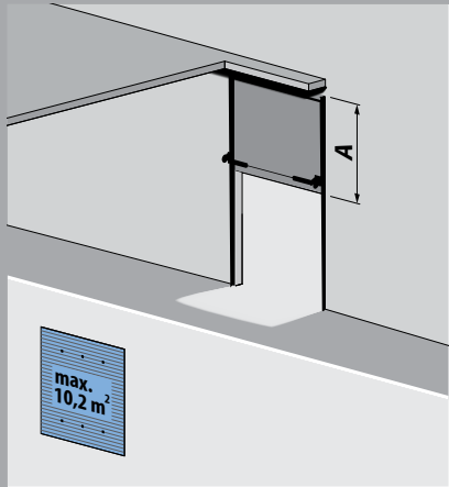
T 500 DS (B550 dock), système de rails vertical avec axe de ressort surbaissé
