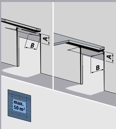
T 400 (B350), système de rails levée semi-verticale
