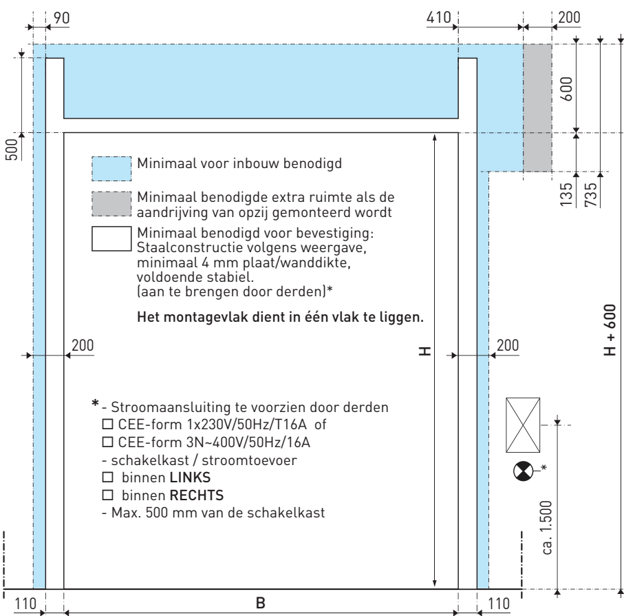
[ Vooraanzicht ]
