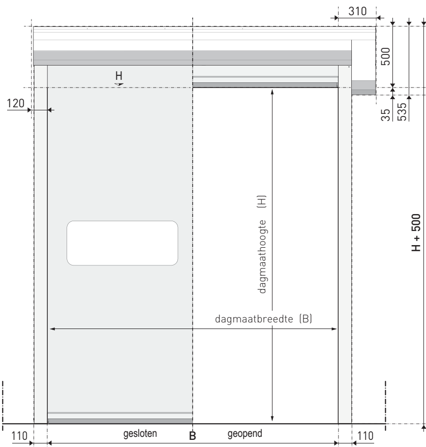
[ Vooraanzicht ]
