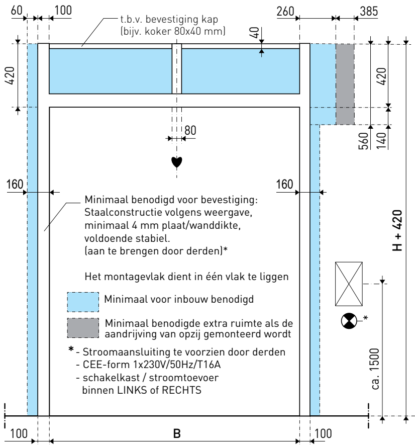
[ Vooraanzicht ]
