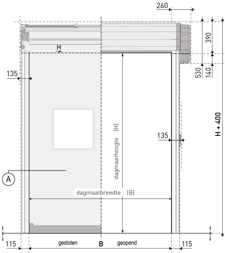
[ Vooraanzicht ]
