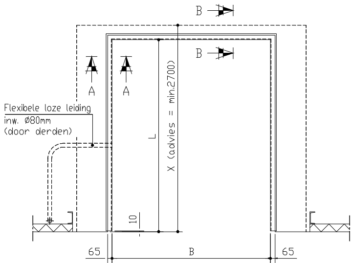
Bovenaanzicht
